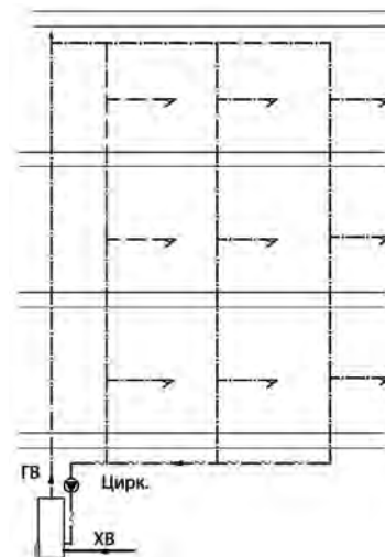
Рис. 7.2. Схема системы ГВС с циркуляцией – верхняя разводка
