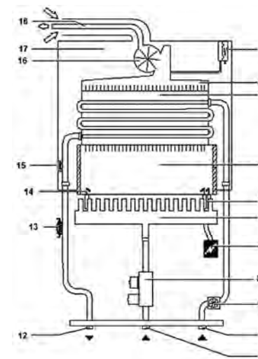
Рис. 10.14. Схема современного газового проточного водоподогревателя [11]: 1 – дифференциальный манометр; 2 – панель камеры сгорания; 3 – теплообменник; 4 – камера сгорания; 5 – электрод поджига; 6 – горелка; 7 – трансформатор поджига; 8 – газовая арматура; 9 – расходомер; 10 – подключение холодной воды; 11 – ввод газа; 12 – подключение горячей воды; 13 – датчик температуры; 14 – ионизационный электрод; 15 – ограничитель температуры; 16 – вентилятор; 17 – камера давления; 18 – коаксиальный дымоход
