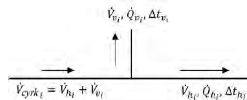
Рис. 9.3. Расчетная схема узла системы ГВС
