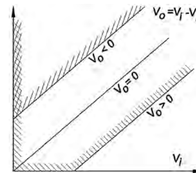
Рис. 3.4. Площадь существования переменной V_0 вместе с пределами и разбиением на площади интегрирования
