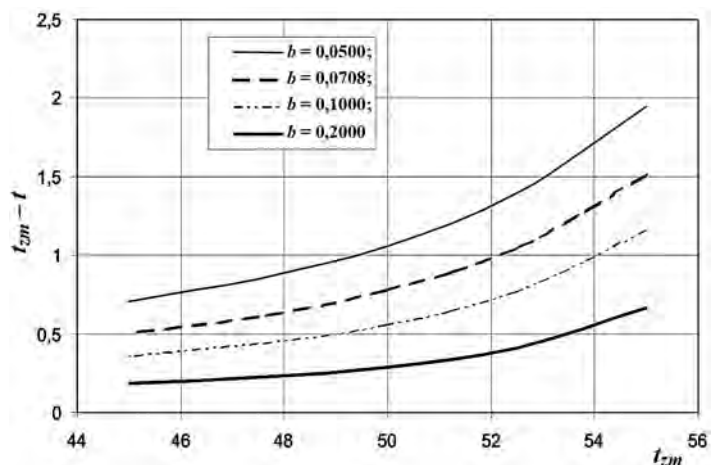
Рис. 8.2. Разница температуры \Delta t_{zm} между температурой закрытия термостатического циркуляционного клапана t_{zm} и температурой в месте его установки в зависимости от температуры t_{zm} при разных показателях b , характеризующих клапан ( k_v = 1,505 \text{ м}^3/\text{ч} ; h_p = 2 \text{ м} ; \dot{Q}_r = 250 \text{ Вт} ; a = 0,3 )
