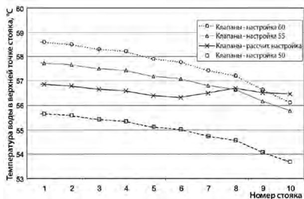
Рис. 9.10. Температура в верхних точках стояков системы из полипропиленовых труб (без теплоизоляции стояков) при расчетных настройках, а также при разных постоянных настройках термостатических циркуляционных клапанов
