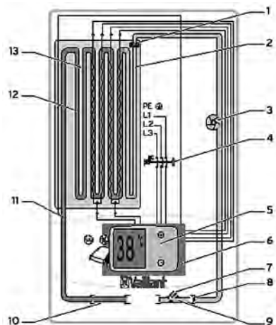
Рис. 10.13. Схема современного электрического проточного водоподогревателя [12]:
