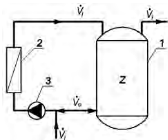
Рис. 10.8. Принципиальная схема проточной системы с насосом и баком-аккумулятором: 1 – бак-аккумулятор; 2 – теплообменник; 3 – насос
