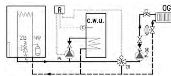
Рис. 11.6. Реализация приоритета приготовления горячей воды с помощью трехходового регулирующего клапана
