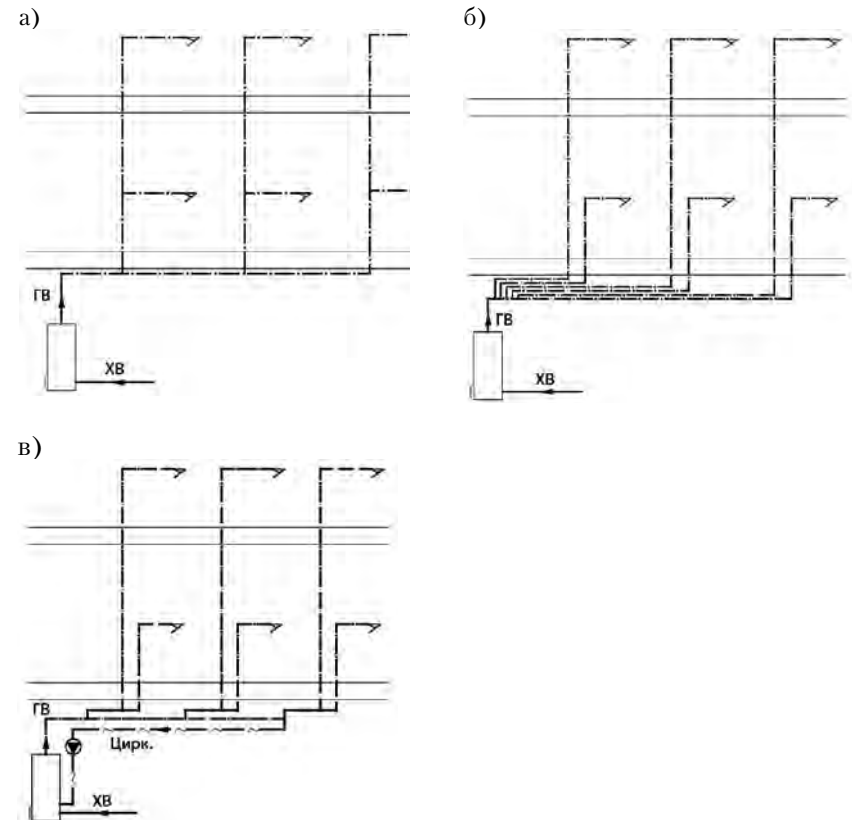
Рис. 7.5. Альтернативные схемы систем ГВС частных домов: а) с подачей горячей воды к водоразборным точкам по стоякам; б) с индивидуальной разводкой к водоразборным точкам; в) с циркуляцией горизонтальных трубопроводов и индивидуальной разводкой к водоразборным точкам
