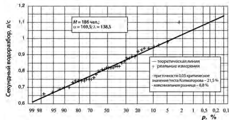
Рис. 2.15. Теоретическая вероятность появления максимального секундного (пятисекундного) потребления в течение суток в соответствии со сложным Пуассоновским процессом и данные натуральных измерений
